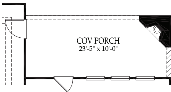
Optional Exterior Fireplace
